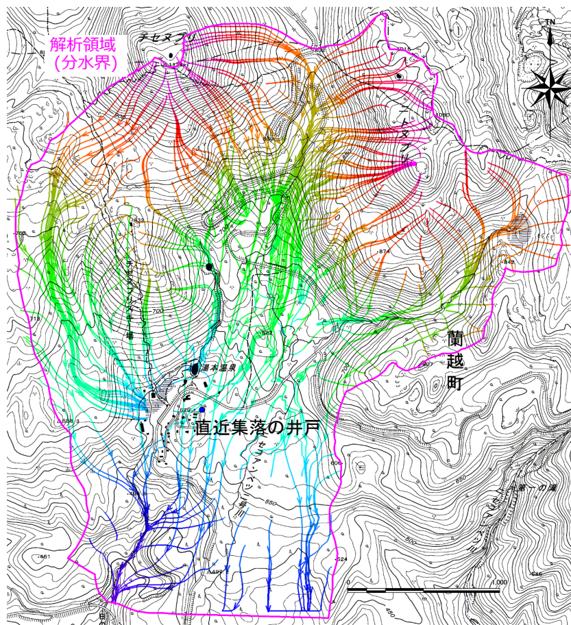
解析領域全体から発生させた流線(平面図)
