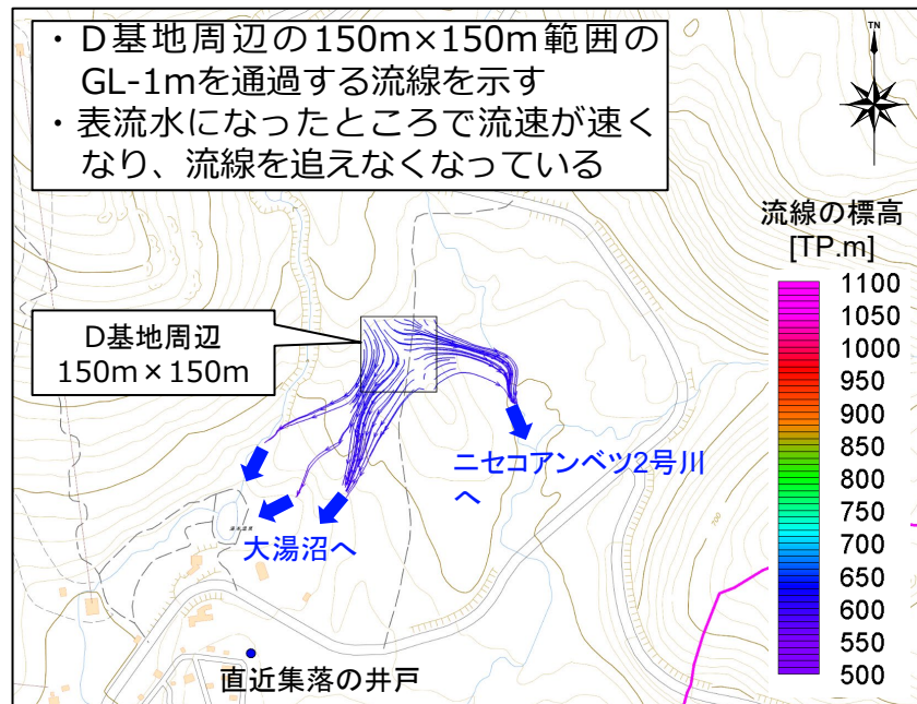
D基地付近から出発する流線
