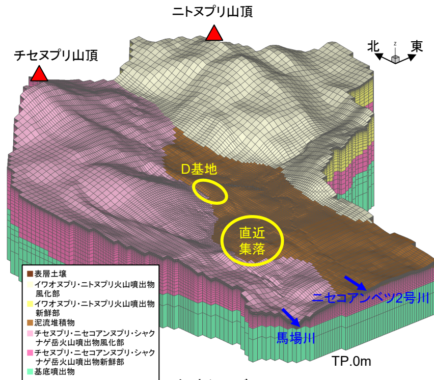
解析モデル
